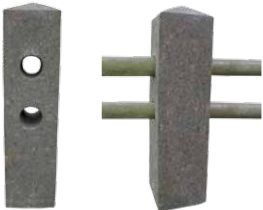
Zaunelement für zwei horizontale Bambusstäbe 1 Zaunelement für zwei horizontale Bambusstäbe, Loch - Ausrichtung 180° - Gerade, 80 cm H | Naturstein (Basanit), Steinmetzarbeit
